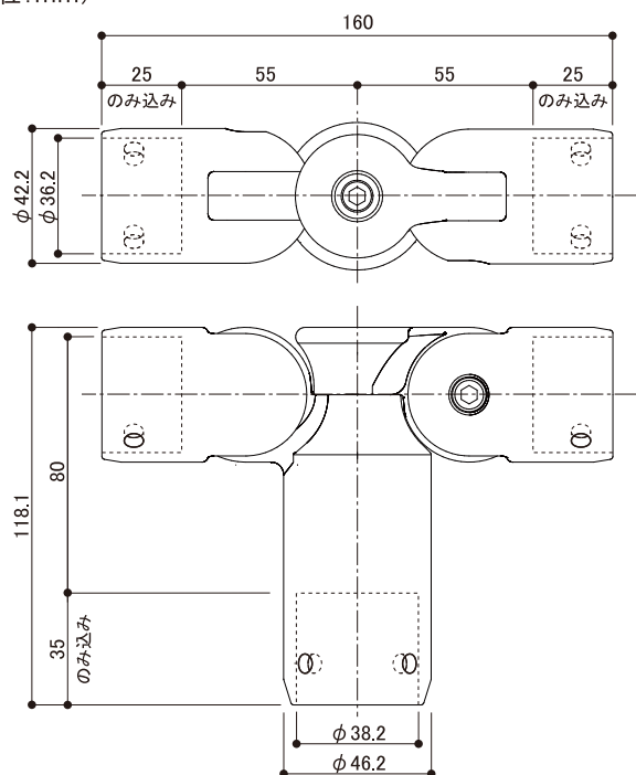
支柱用コーナージョイントN本体 【数量】1個 【材質】アルミ合金
