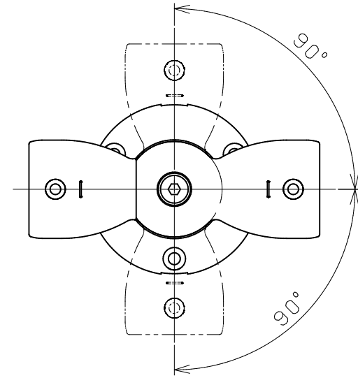
角度調整範囲図 (S=1/2)
