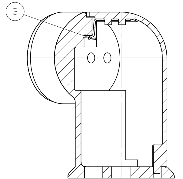
A-A断面図 尺度(1/1)
