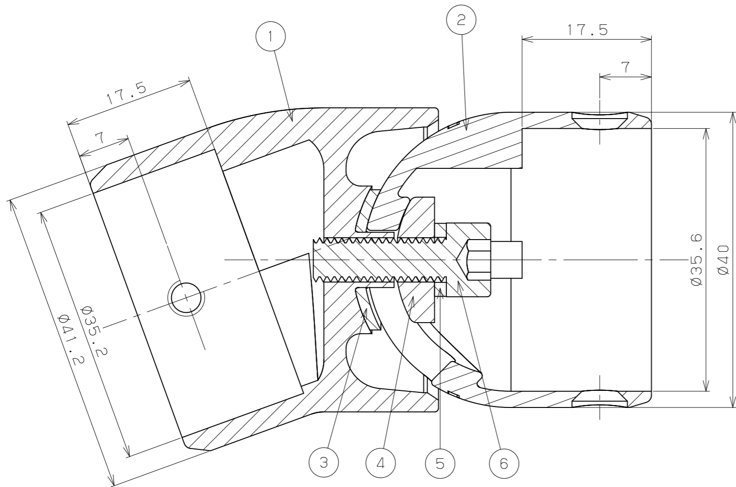
A-A 断面図 (S=2/1)
