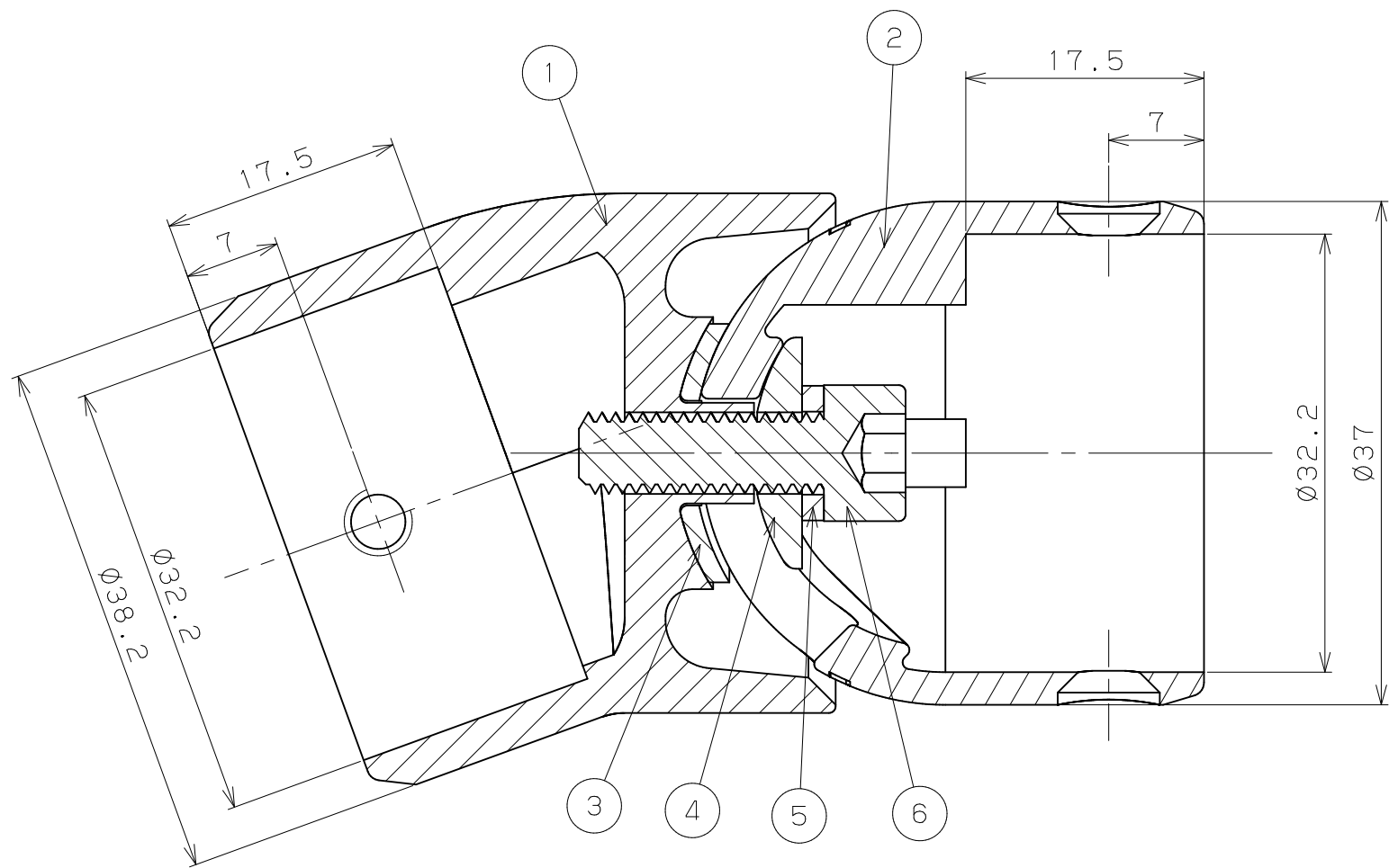
A-A断面図 (S=2/1)
