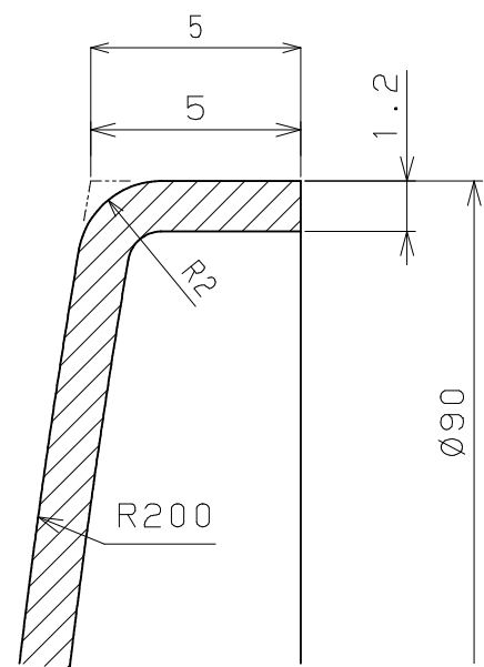
A-A断面図 S=5/1
