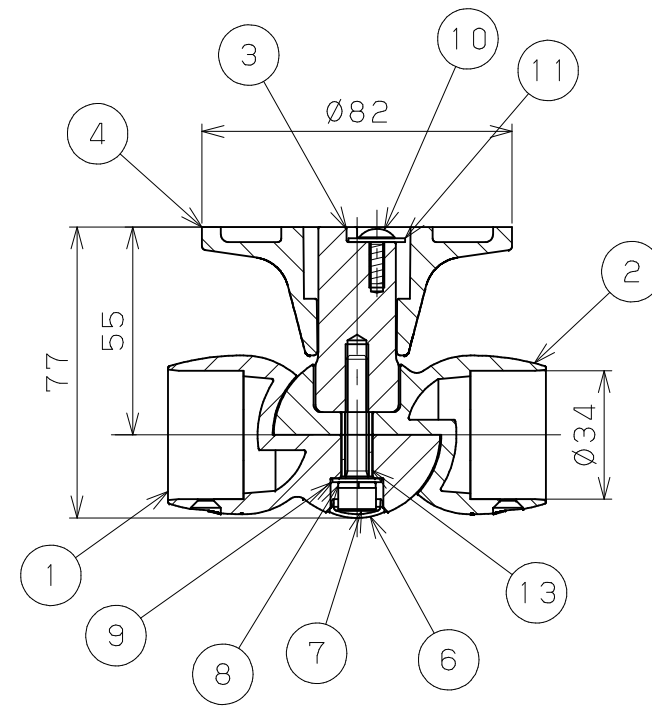
A-A断面図
