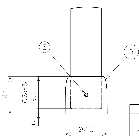
B部詳細図 S=1/2 (床側：Nエンドソケット)
