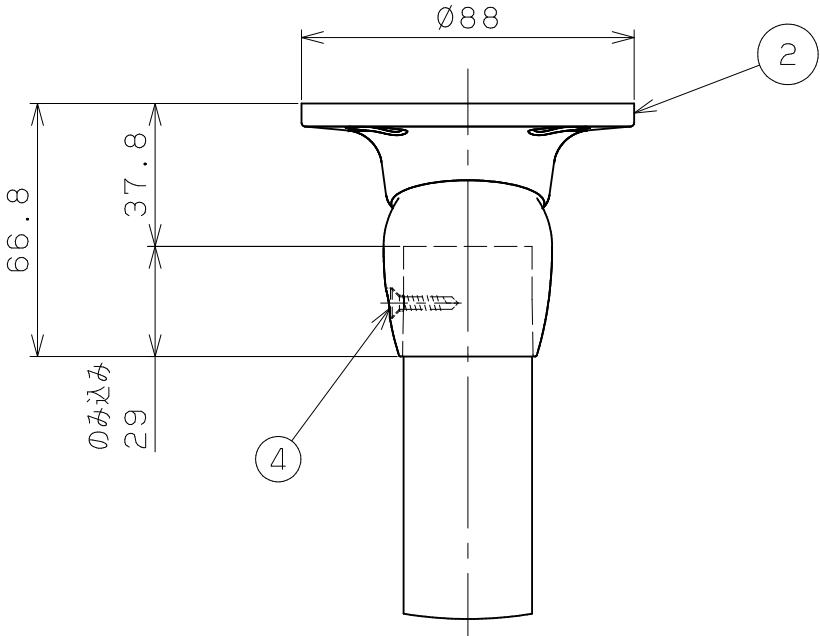
A部詳細図 S=1/2 (天井側：自在ソケット)
