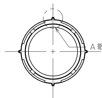
C-C矢視 リップ詳細
