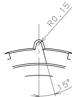
A部詳細 S=4/1
