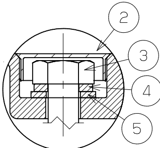
キャップ納まり図
