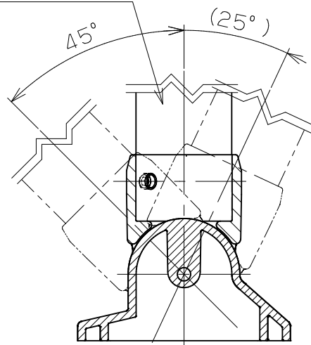
B-B断面図 (S=1/2)
