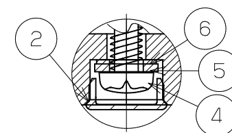
キャップ納まり図
