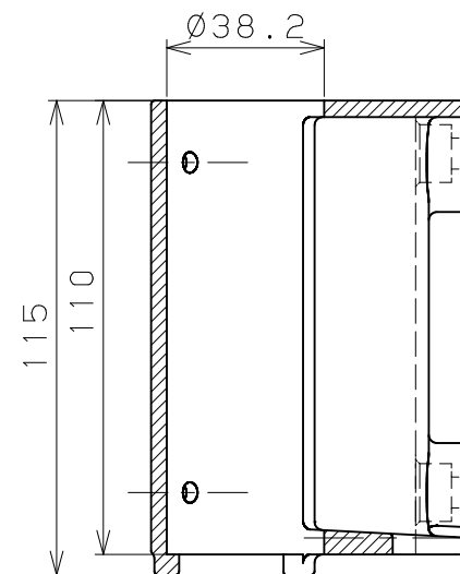
A-A断面図
