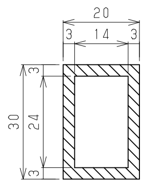
支柱埋め込み部断面寸法 S=1/1
