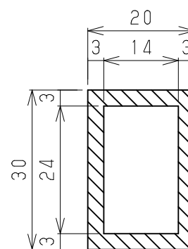
支柱埋め込み部断面寸法 S = 1 / 1
